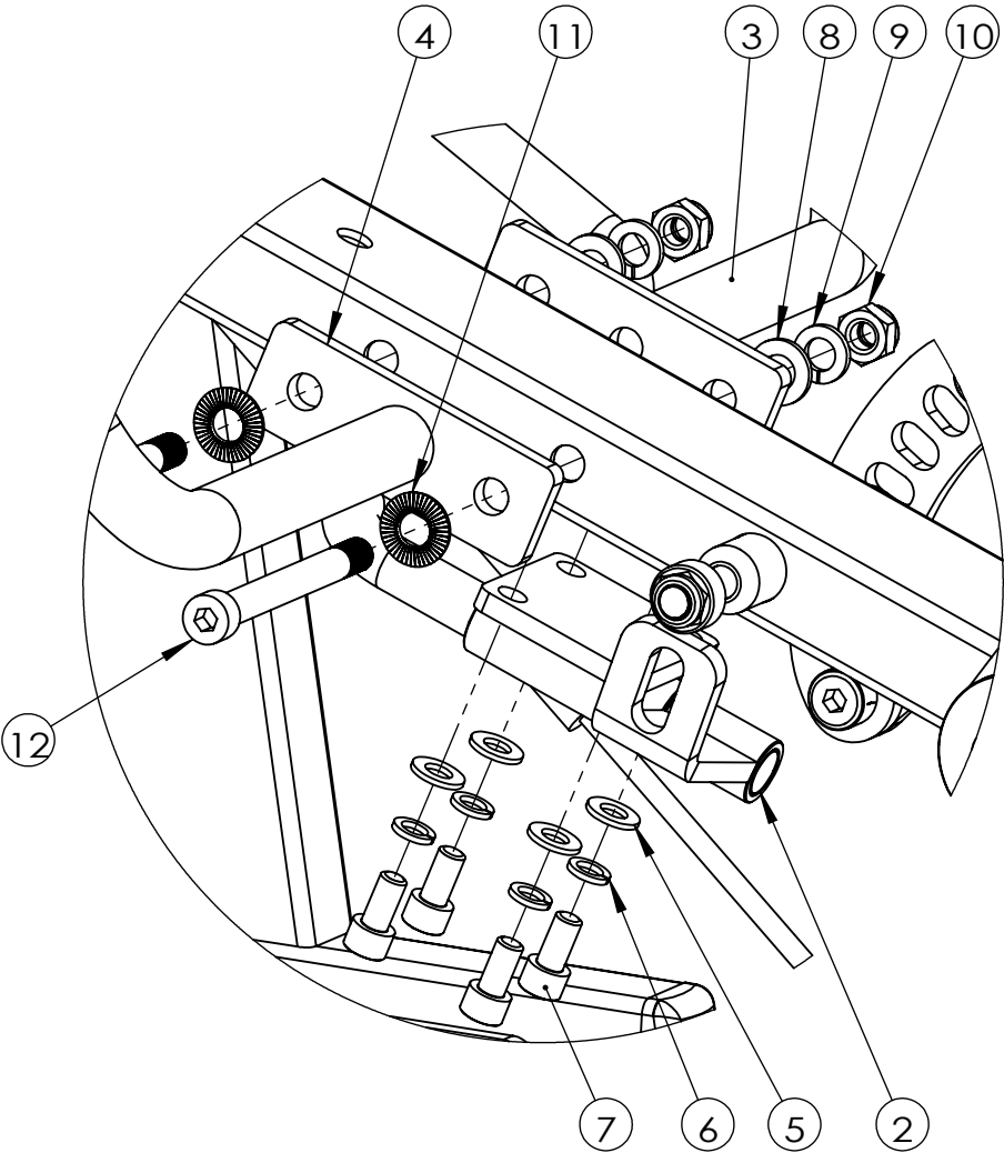
局部视图 A 比例 1 : 3
